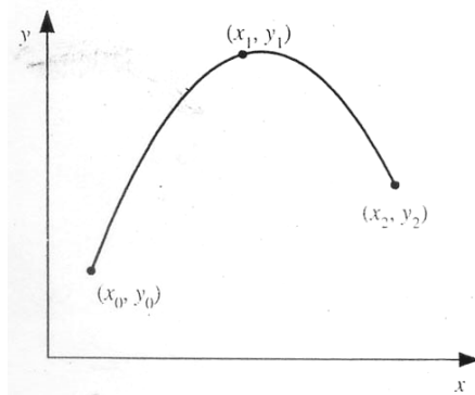
Gambar 3.3. Interpolasi Kuadratik
