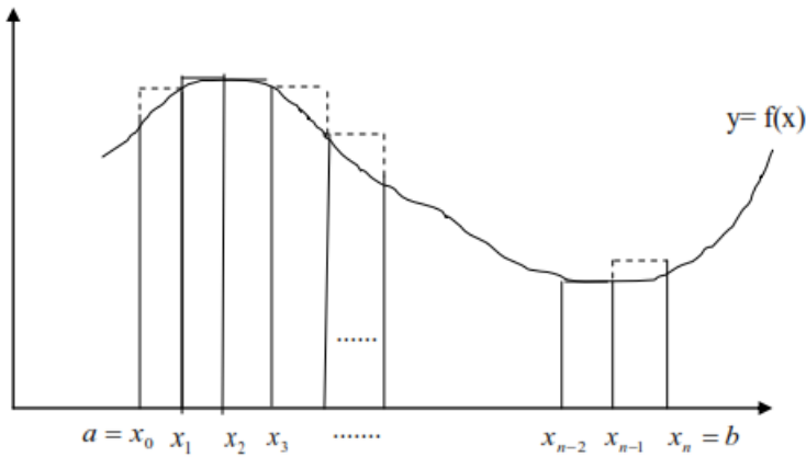
Gambar 4.3 Kaidah segiempat gabungan
