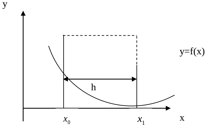
Gambar 4.2 Kaidah Segiempat
