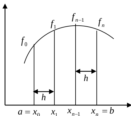
Gambar 4.1 Metode pias
