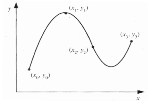
Gambar 3.4. Interpolasi Kubik
