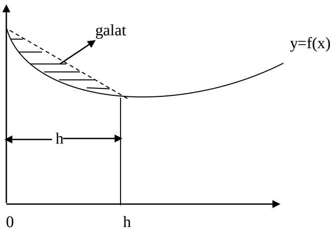
Gambar 4.5 Galat Kaidah Trapesium (yang diarsir)
